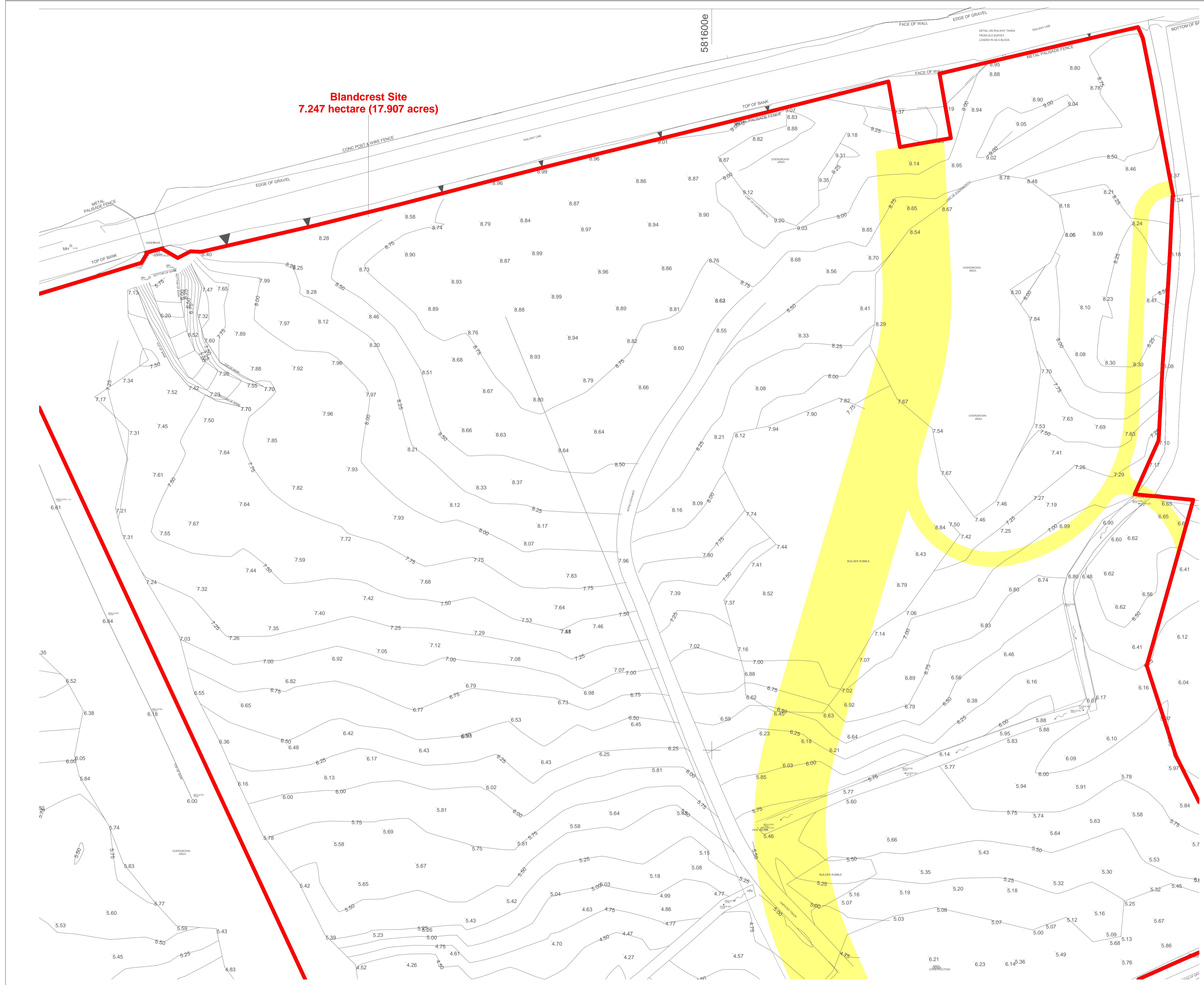
1 Existing Site Survey 05 1 : 500
